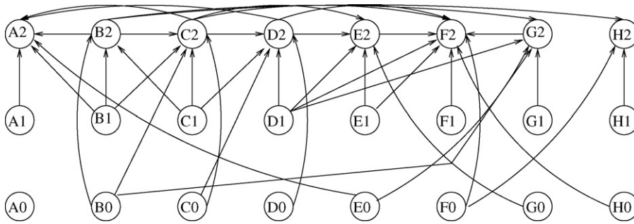
Fig. 4. Best model.
